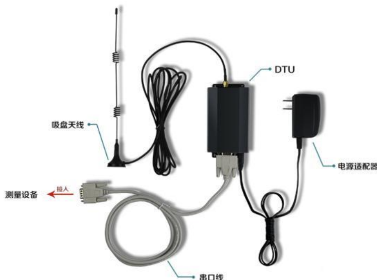
图 7-14 DTU-无线短信报警器
