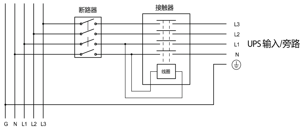
三相输入系统示意图
