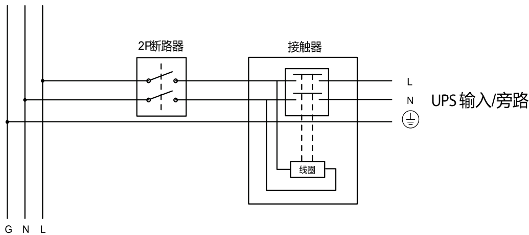
单相输入系统示意图
