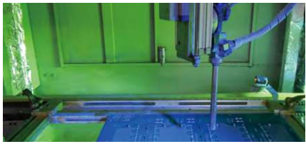
PCBA喷涂后蓝光检测
