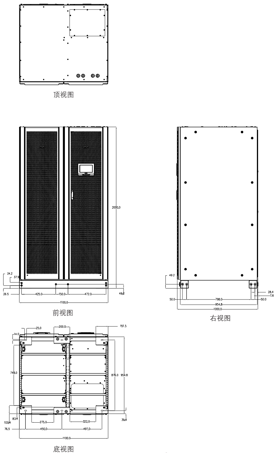
图3-2: UPS 尺寸
