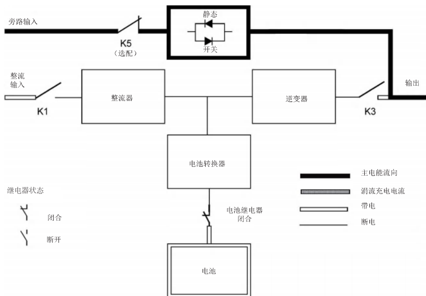
图2-7：旁路模式电能通过 UPS 的路径
