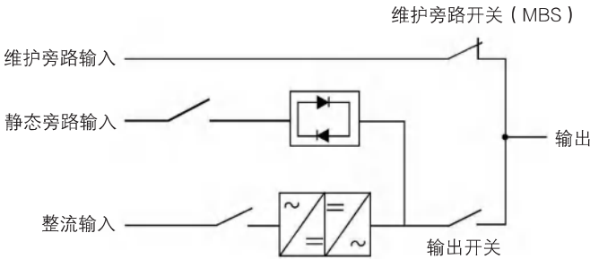
图6-39: 维护旁路模式下开关状态
