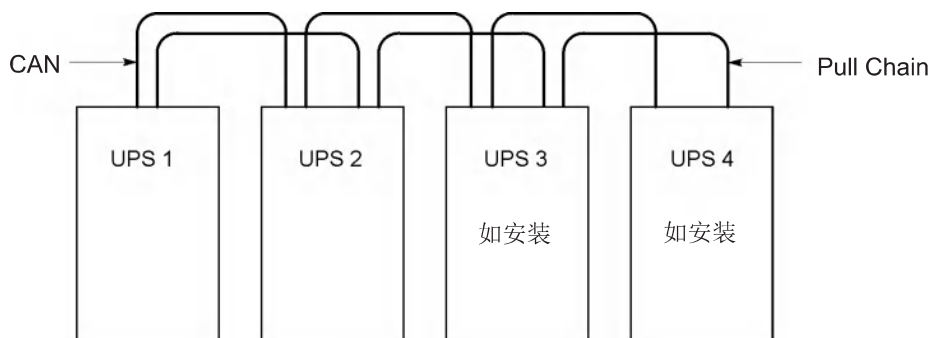
图4-11：并机UPS系统的CAN和Pull-Chain的简化配线
