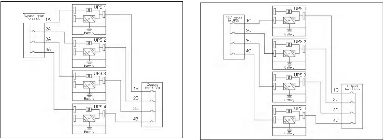
并机系统接线图
