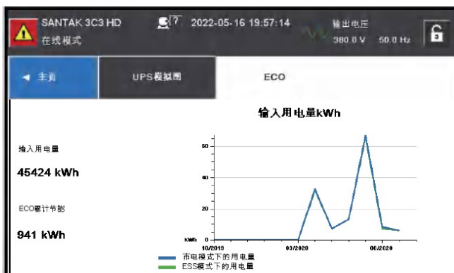
图6-29：ECO屏幕
