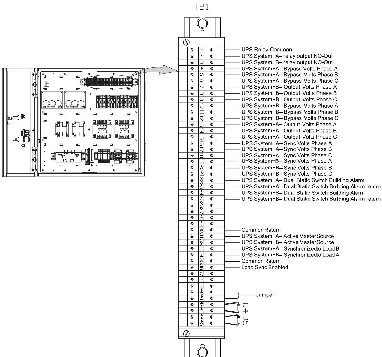
图4-13: 同步盒 TB1 端子位置
