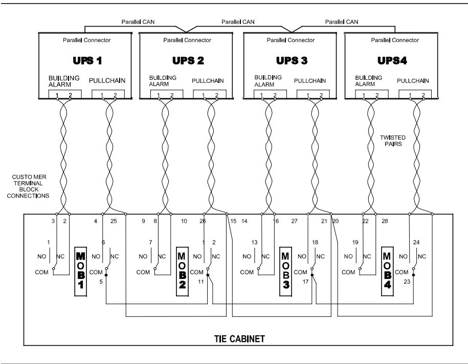
并机信号线和CAN通讯控制线接线图--带并机柜
