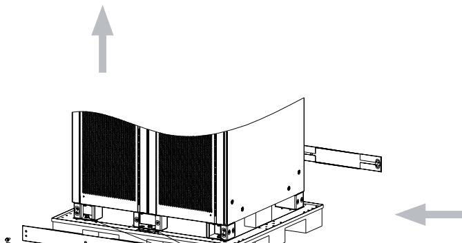
图4-4: 拆除固定螺钉
