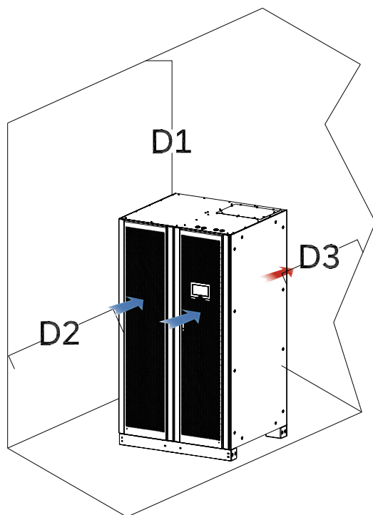
图3-1：UPS 机柜预留空间
