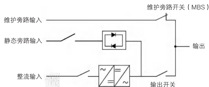
图6-40: 维护旁路模式下开关状态
