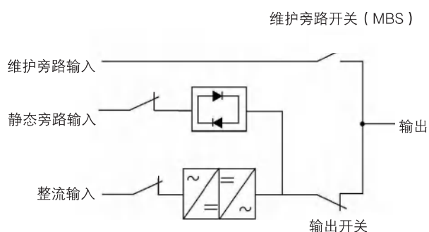
图6-41: 在线模式下开关状态
