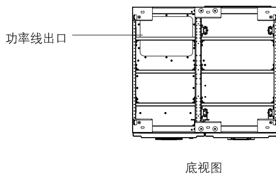
图4-6: 盖板和连接端子位置
