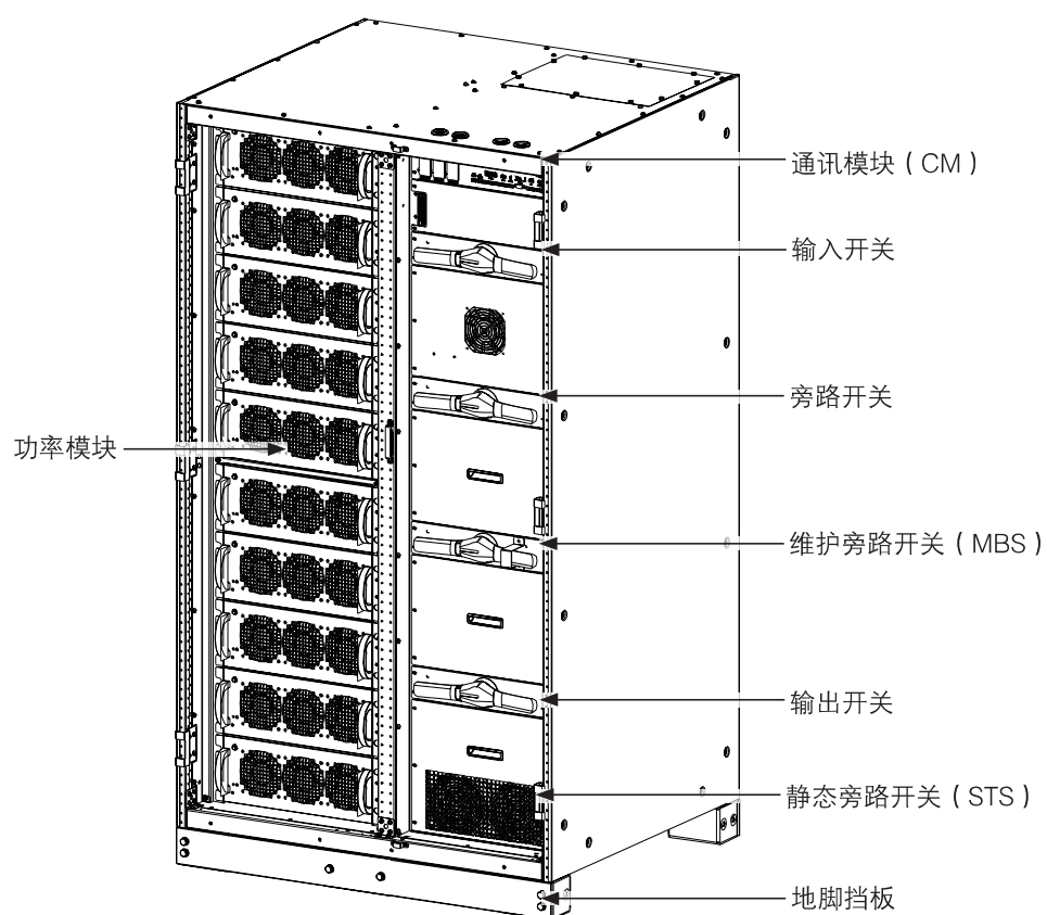
图2-2: 产品结构图
