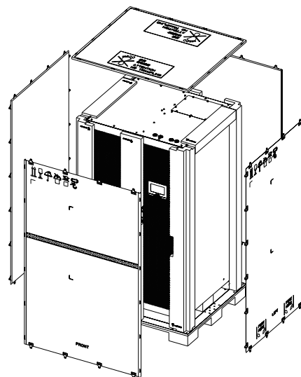
图4-2: 移除木箱
