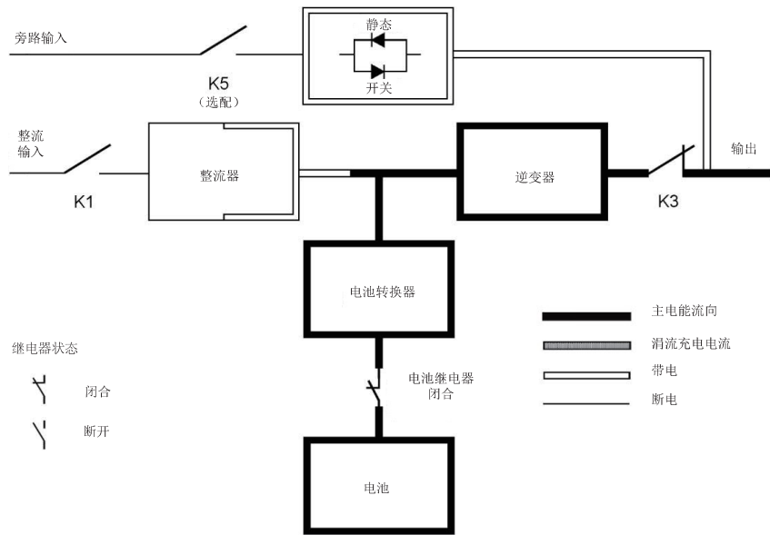
图2-6: 电池模式下电能通过 UPS 的路径
