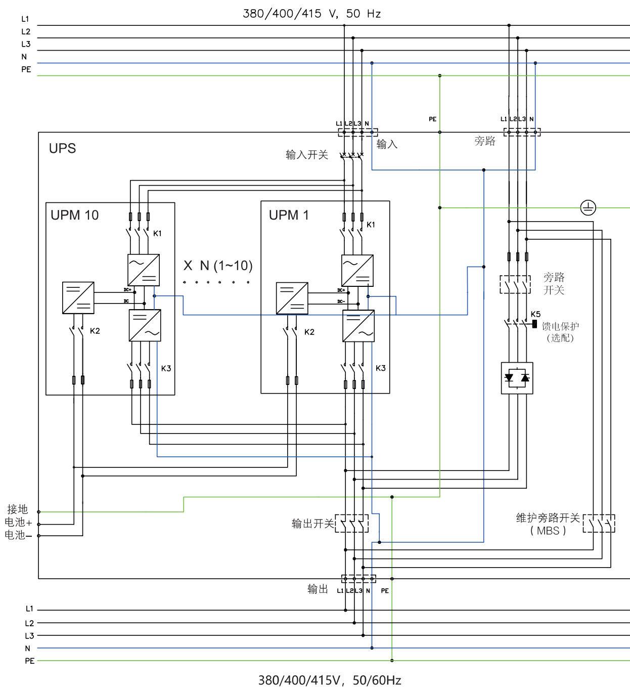
图2-3: UPS 线路图
