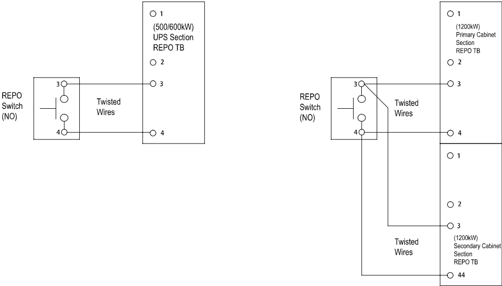
图4-8：常开 REPO 开关配线
