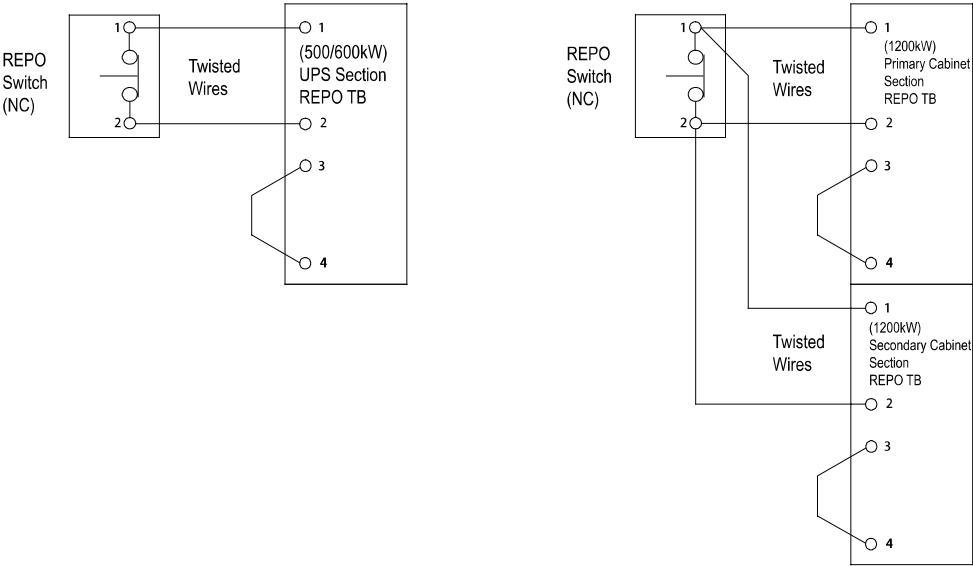
图4-9：常闭REPO 开关配线
