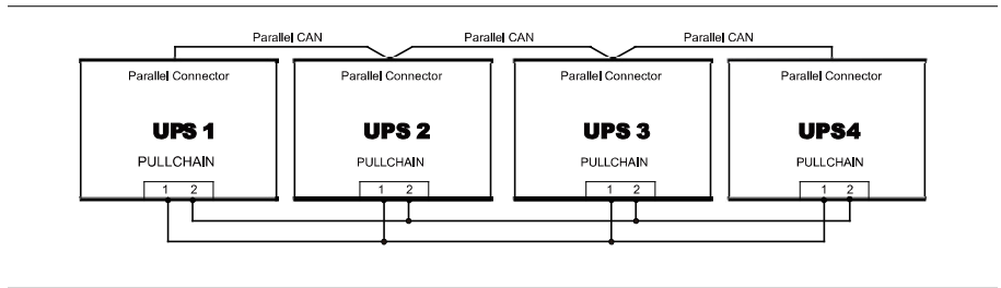
并机信号线和CAN通讯控制线接线图--不带并机柜
