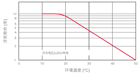
浮充寿命曲线
