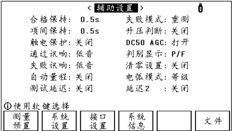
图 4-4 测量配置页面
