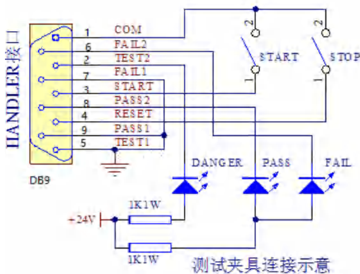
HANDLER 外部电路连接示意图（外接电源）
