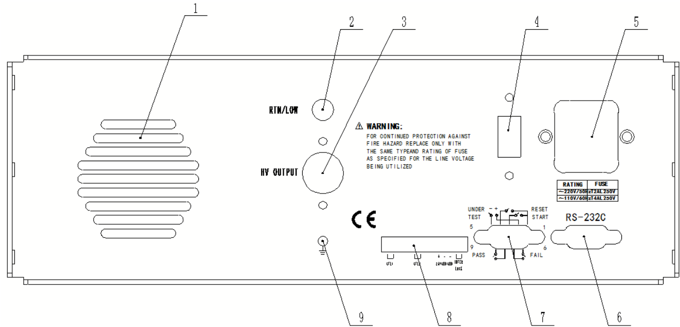
图 3-2 后面板说明
