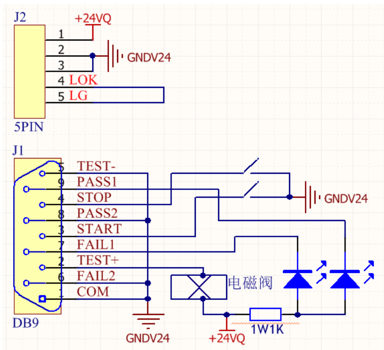
外部电磁阀连接示意图
