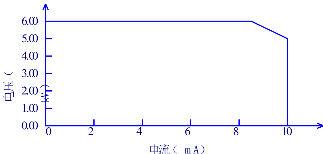
图 3-4 直流电压输出范围
