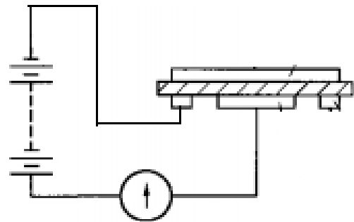
b)测量表面电阻率线路
