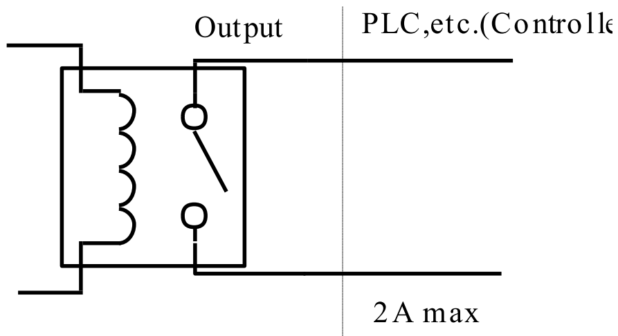
输出端原理图
