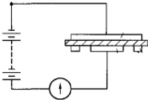
a)测量体积电阻率线路
