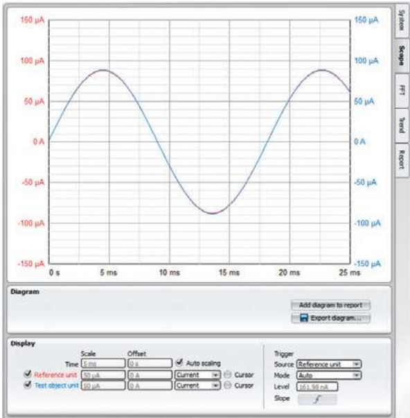
示波器视图
