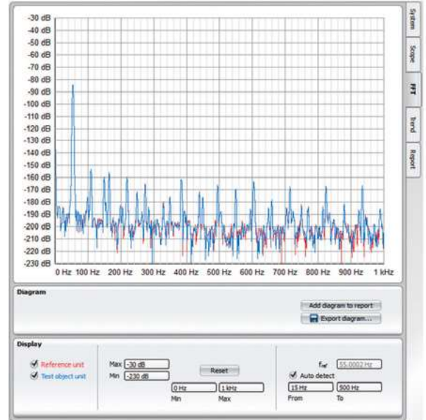
FFT 视图
