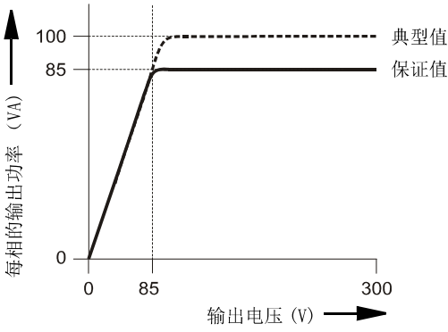
三相工作的功率图
