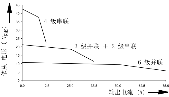
典型依从电压 (50/60 Hz)
