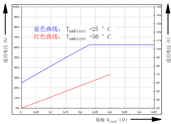
保证连续运行的典型允许依从电压
