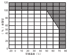
图3: 输出降额曲线图(全范围)
