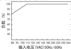
图3: 输出降额曲线图(全范围)
