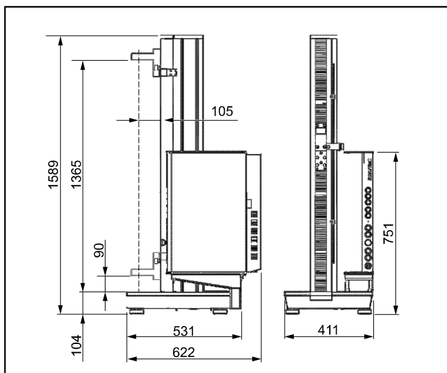
Maße Prüfsystem TH
