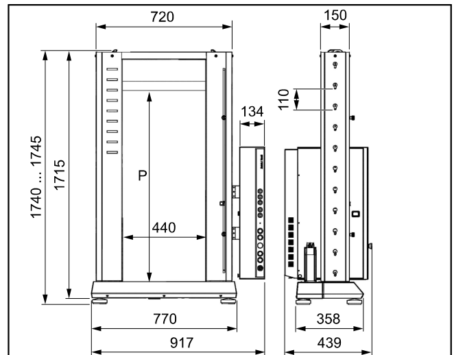
ProLine Z005 und Z010 TH, Maße
