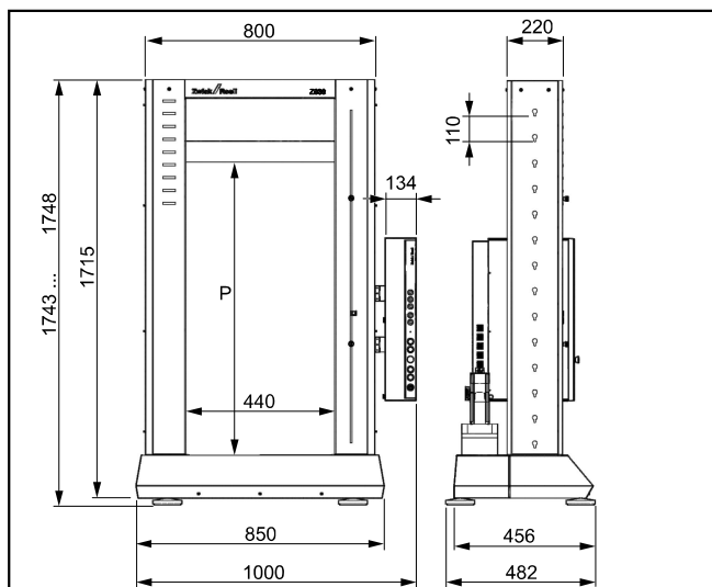
ProLine Z030 und Z050 TN, Maße
