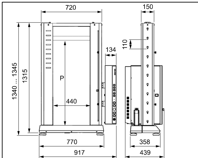
ProLine Z005 TN, Z010 TN und Z020 TN, Maße
