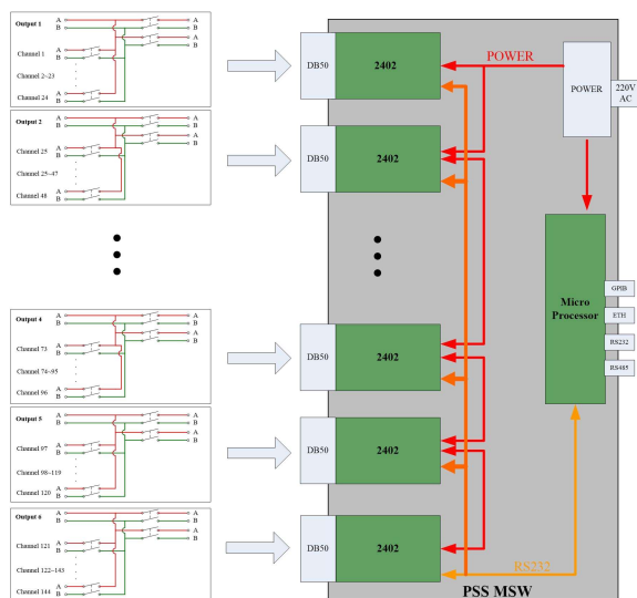
电开关主机框图
