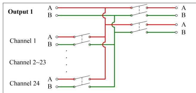
2402 矩阵开关卡
