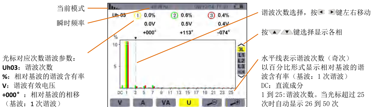
图 7-8 线电压谐波 3L 显示
