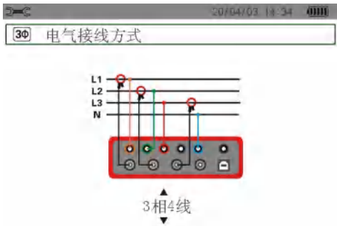
图 4-6 三相 4 线连接
