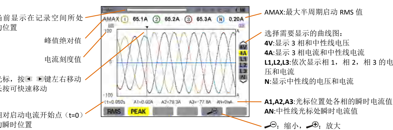
图 6-11 4A 峰值显示屏幕
