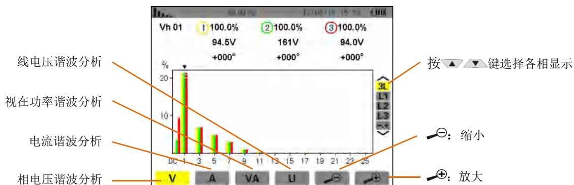
图 7-1 谐波模式屏幕
