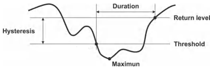
图 17-2 骤降侦测回差图例
