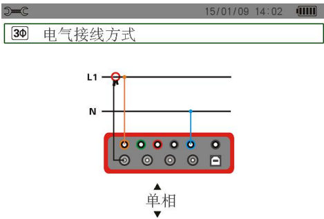
图 4-4 单相连接
