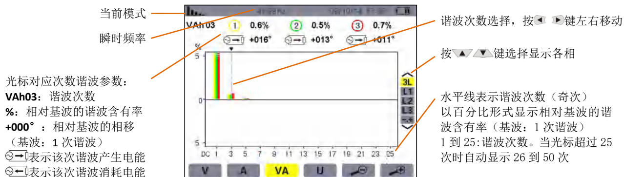
图 7-6 视在功率谐波 3L 显示
