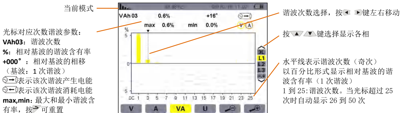
图 7-7 视在功率谐波 L1 显示
