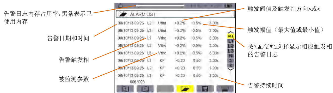
图 9-4 告警日志显示屏
