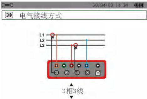
图 4-5 三相 3 线连接
