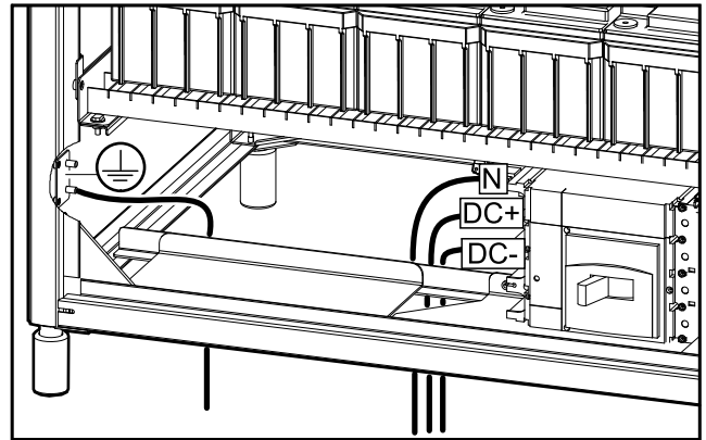
1000 mm 宽标准电池柜
