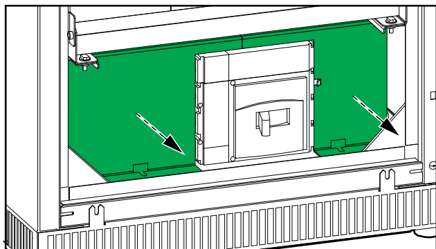
700 mm 宽标准电池柜
