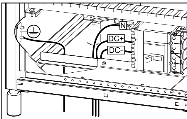
700 mm 宽标准电池柜
