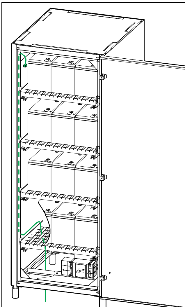
700 mm 宽标准电池柜
