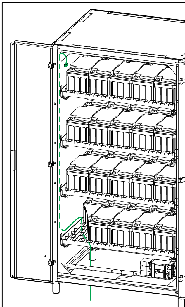
1000 mm 宽标准电池柜
