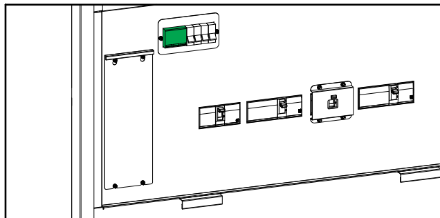
100-120 kVA 384 VDC 3:3 UPS
