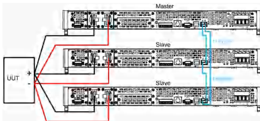
图 6-1 线路连接图
