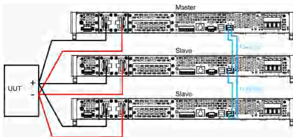
图 5-1 线路连接图
