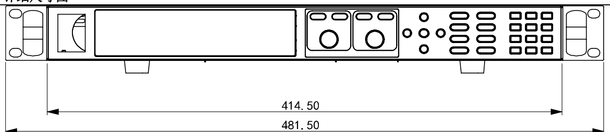
详细尺寸图
