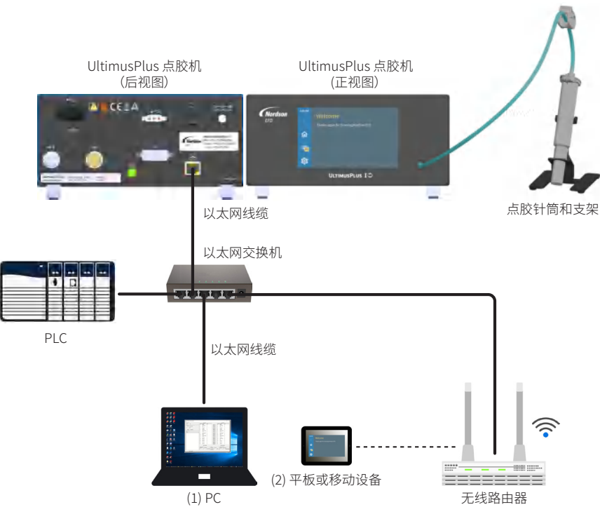
UltimusPlus-NX 点胶机连接的设置示例: (1) 在一台电脑上开启诺信NX客户端应用程序 (2) 在一台平板或移动设备上打开NX网页界面
