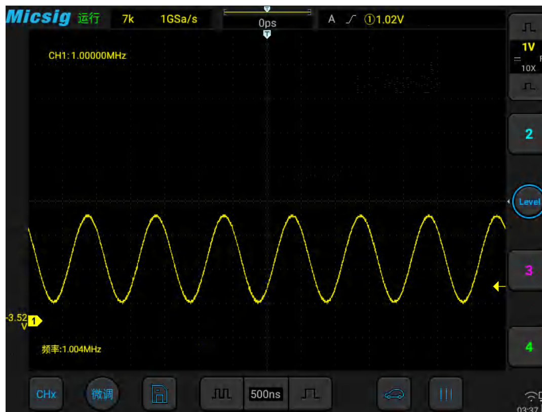
图8-9 频率计测量
