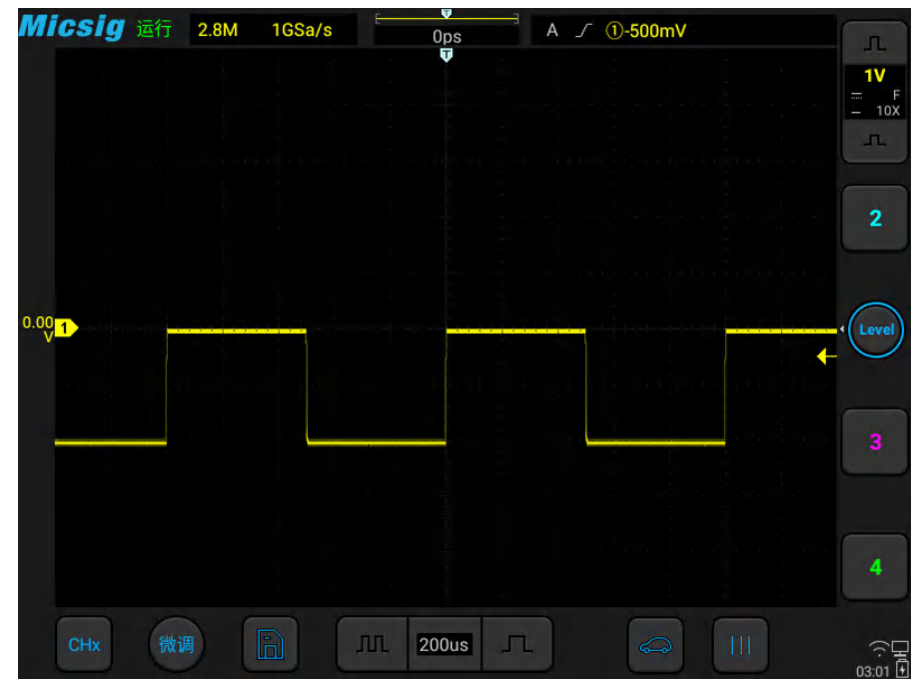
图6-12 反相后
