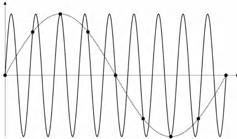
图12-1 混叠
