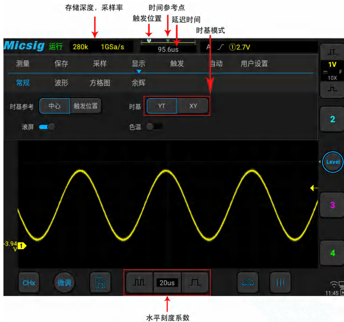
图5-1 水平系统
