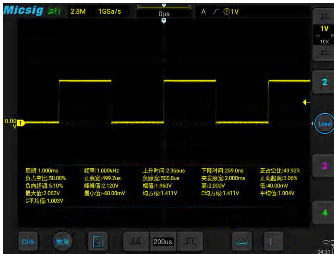
图8-3 全部测量
