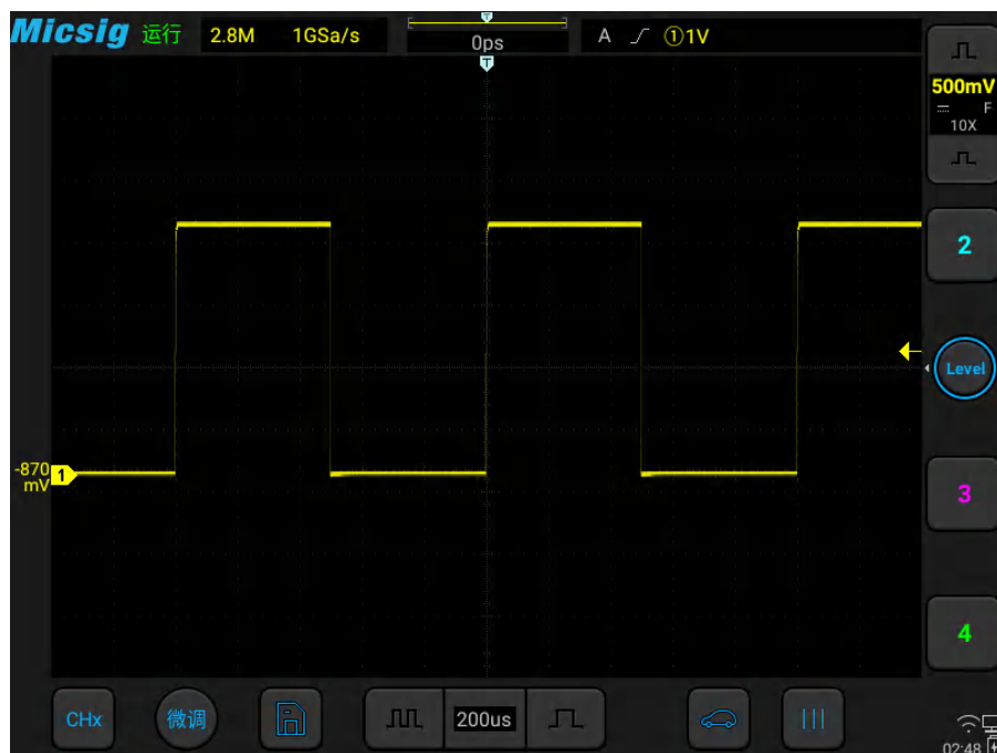
图6-7 DC耦合
