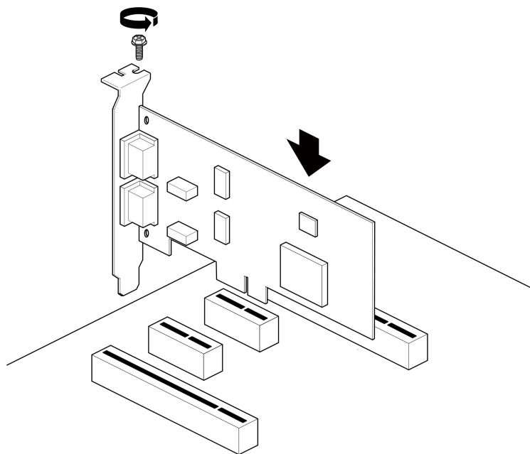
图 2.3 PCIe-9120I 系列工业级 CAN 接口卡
