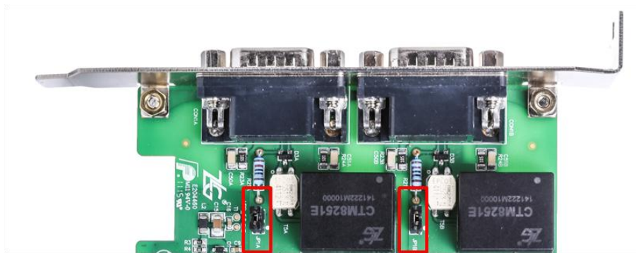
图 2.2 终端电阻选择示意图
