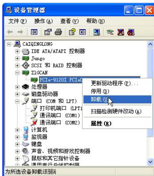
图 3.8 卸载驱动
