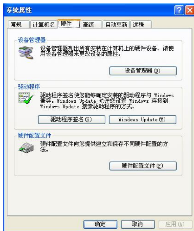
图 3.7 系统属性
