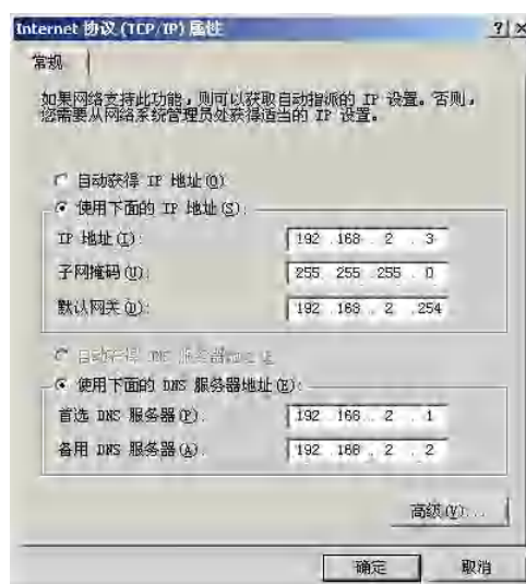
图 5.7 TCP/IP 属性
