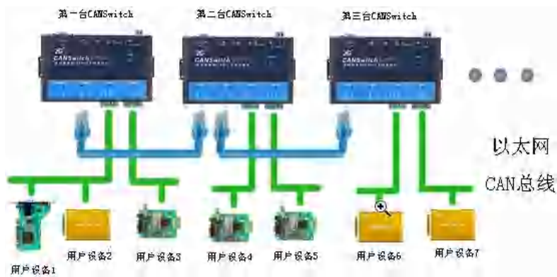
图 3.3 Hub 模式下系统框图
