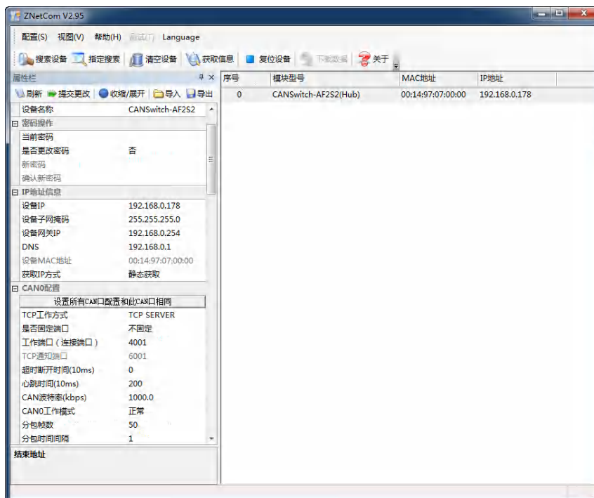
图 5.11 CANSwitch-AF2S2 设备配置信息集线器（Hub）模式
