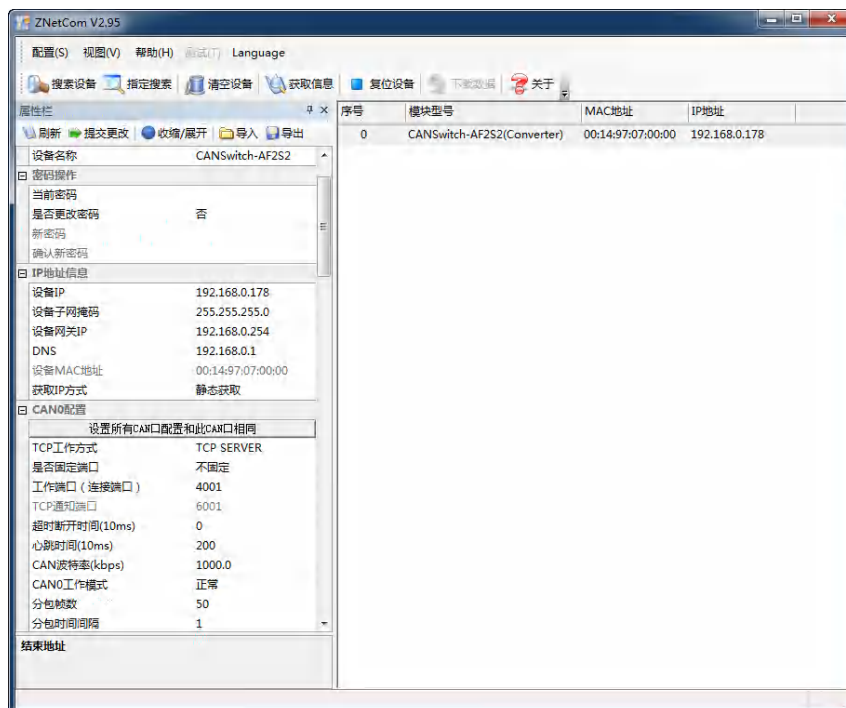
图 5.12 CANSwitch-AF2S2 设备配置信息转换器（Converter）模式
