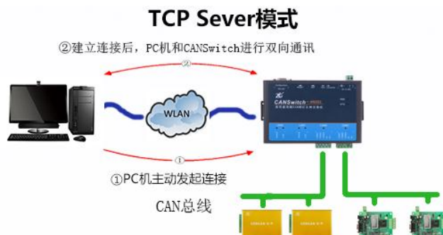
图 4.11 TCP Sever 模式通讯示意图
