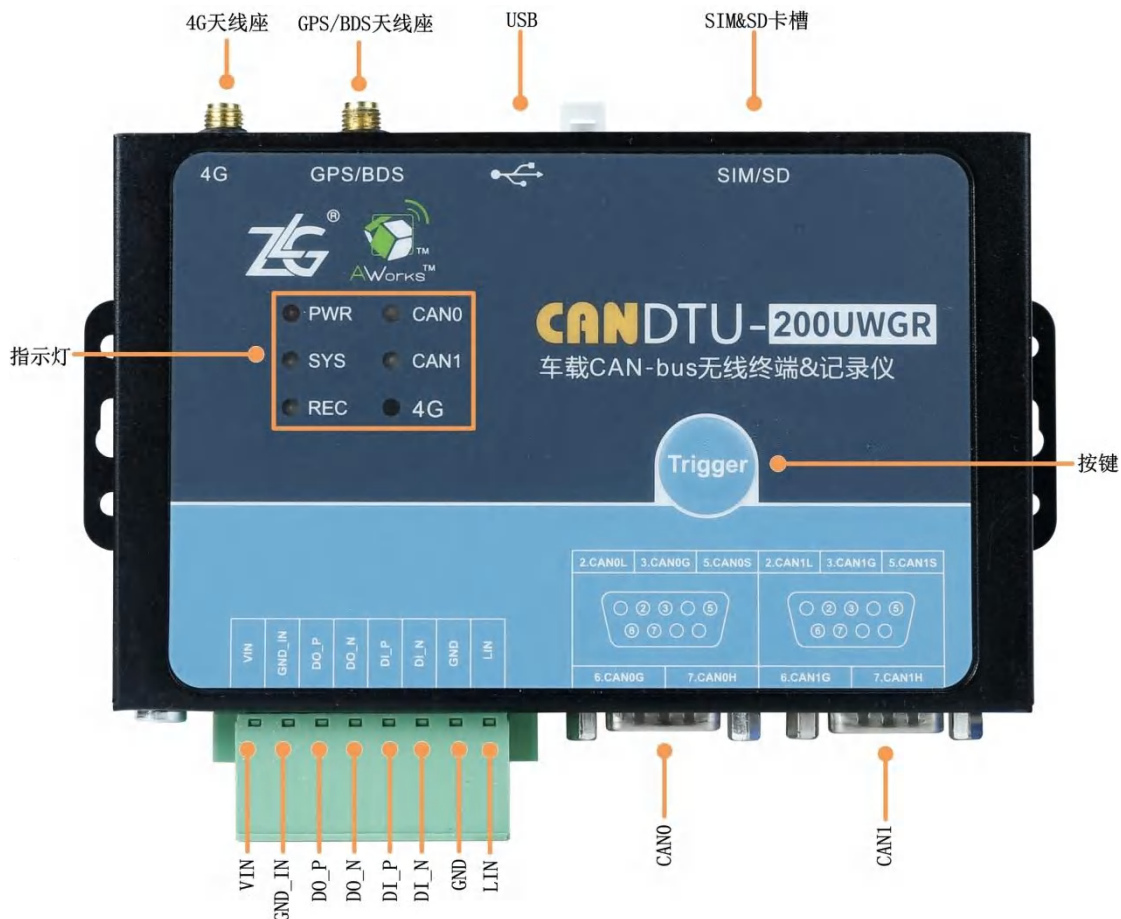
图 3.1 面板布局
