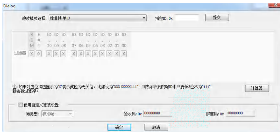
图 4.16 滤波计算器
