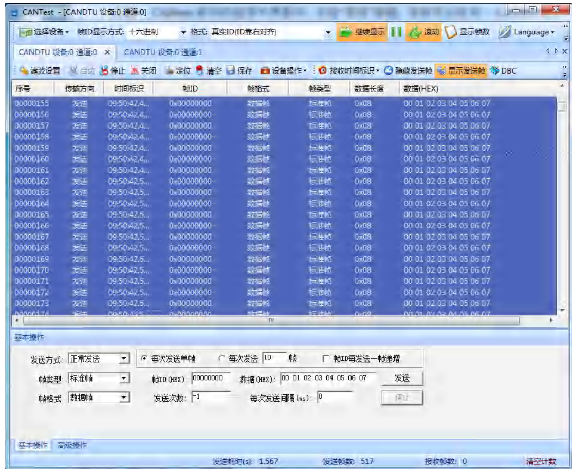
图 5.8 CANDTU-200UR 双路 CAN 之间通信
