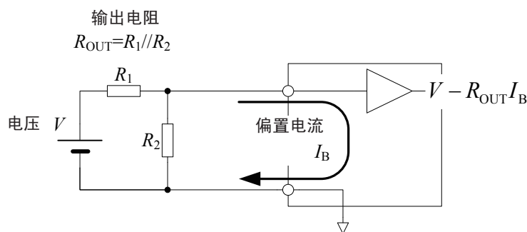
图 偏置电流的影响
