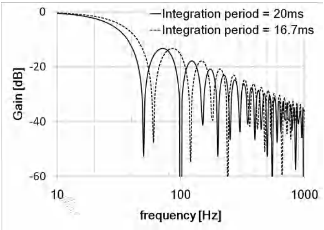
图6 通过积分除去噪音的特性
