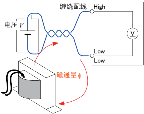
图4 缠绕配线的降噪措施
