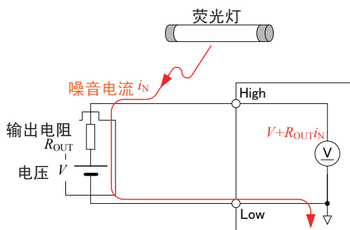
图1 与高电压线路的噪音耦合
