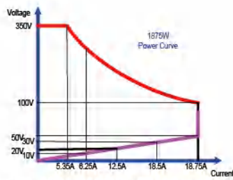
AEL-5002-350-18.75功率曲线图
