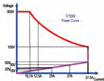
AEL-5004-350-37.5功率曲线图
