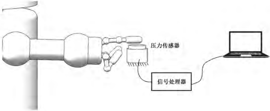
图 6 手指指力测试示意图
