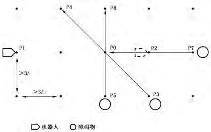
图 5 障碍物规避测试示意图
