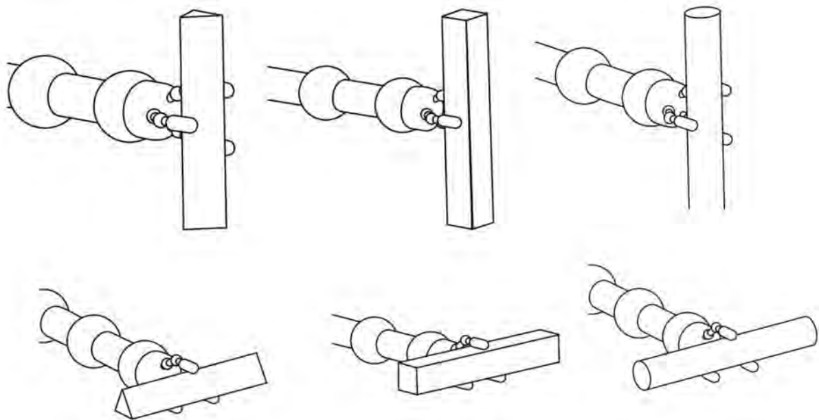
图 7 手臂负载能力测试示意图
