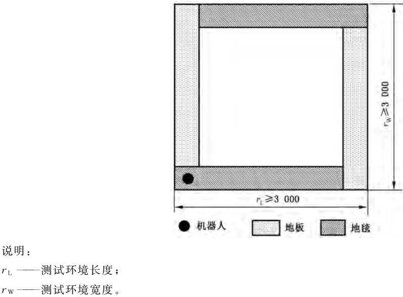
图 8 持续工作时间测试环境
