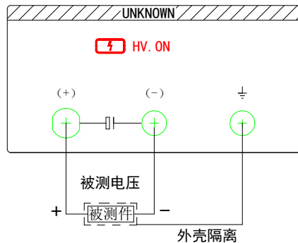
图 3-7 测试连接图
