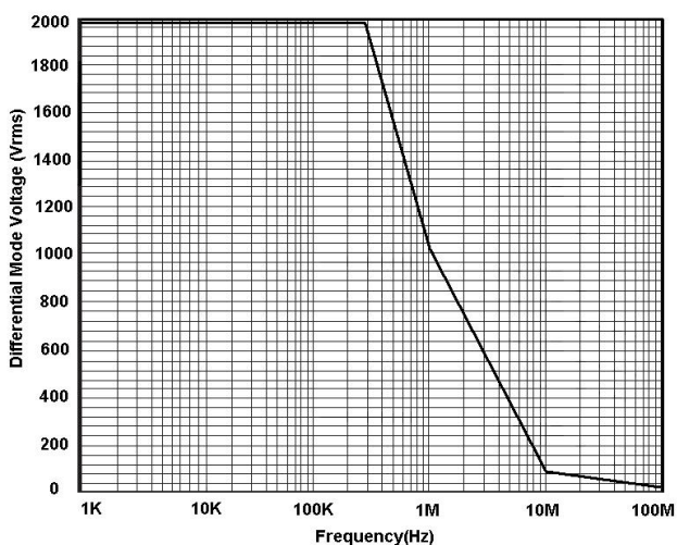
图 3: DP6280D 最大差模电压 VS 频率
