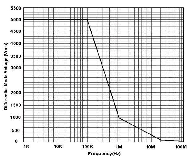
图 4: DP6700D 最大差模电压 VS 频率
