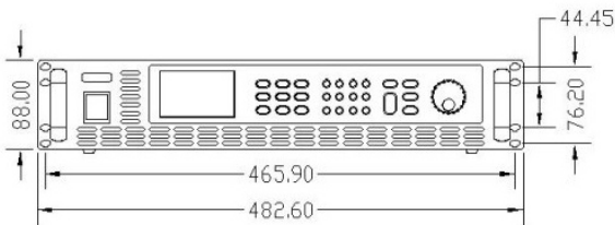
2U机型尺寸图
