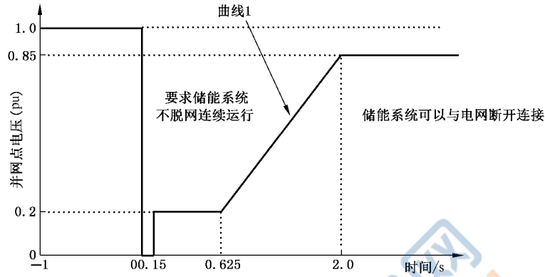
图 4 低电压穿越曲线
