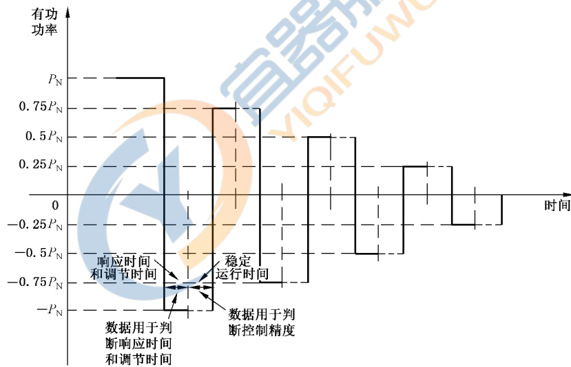
图 2 升功率测试曲线
