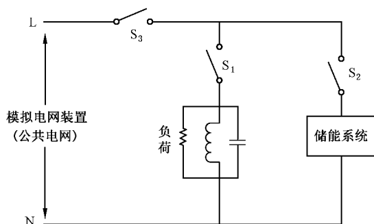
图 6 非计划孤岛保护功能测试
