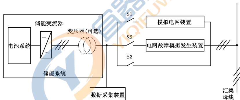
图 1 储能系统测试接线示意图
