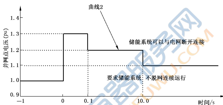
图 5 高电压穿越曲线
