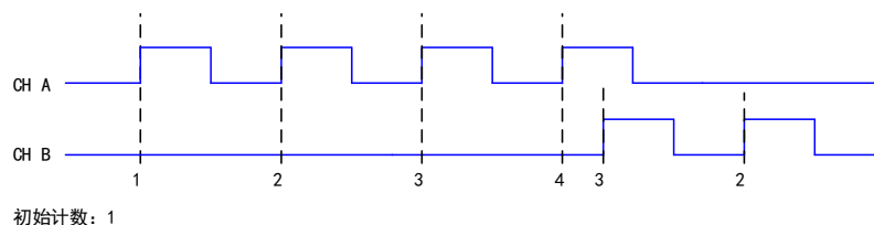
图 6-7-4 双脉冲编码
