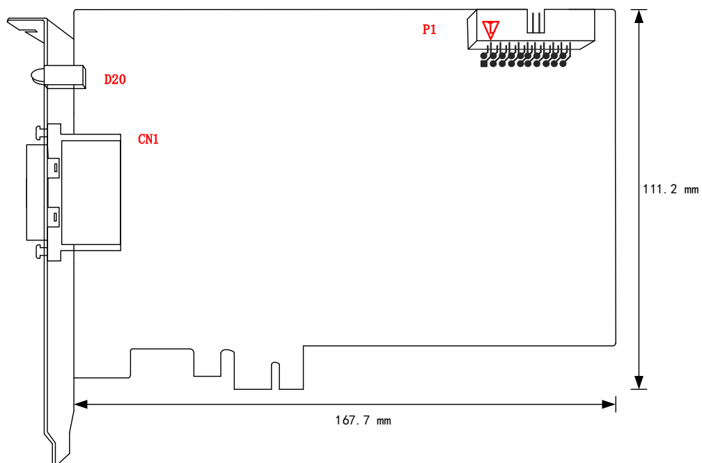
图 3-2-2 PCIE 978X (A_B)板卡尺寸图
