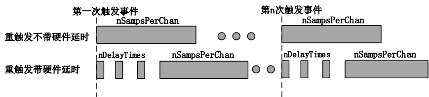
图 8-2-4 重触发
