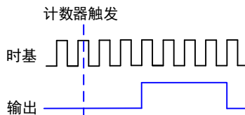
图 6-8-1 单脉冲生成
