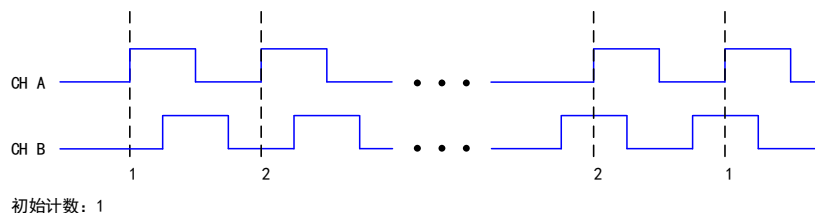
图 6-7-1 X1 编码
