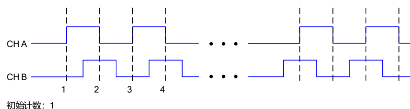
图 6-7-2 X2 编码
