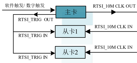
图 4-9-3 采用 RTSI_TRIG 触发主从卡同步的级联方式
