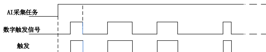
图8-3-9 数字边沿触发--下降沿触发
