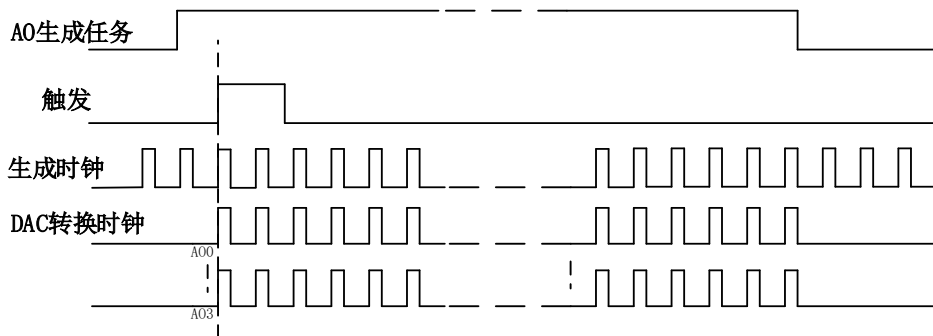
图5-7-3 内、外时钟连续生成
