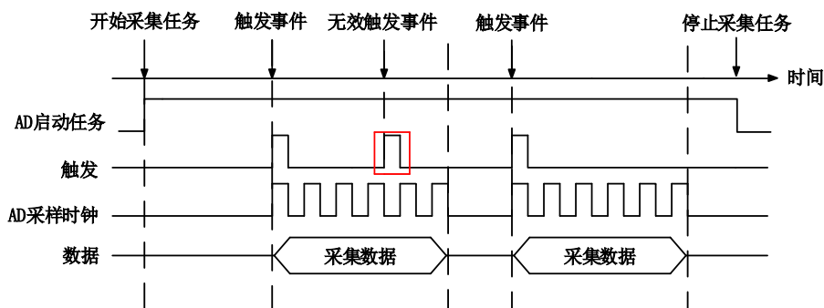
图 8-2-5 上升沿重触发
