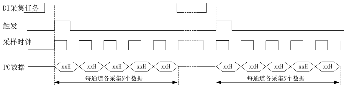
图 7-5-2 有限点采样
