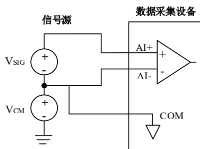
图 4-4-1 AI 信号正确的连接示意图
