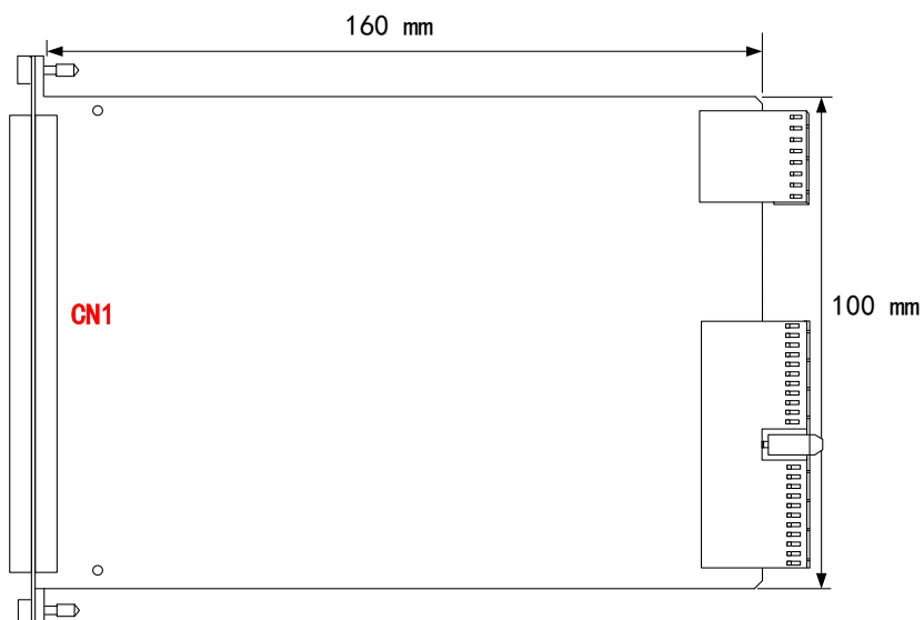
图 3-2-1 板卡尺寸图
