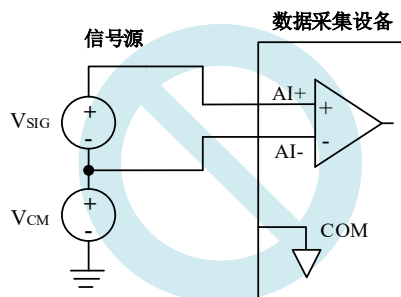
图 4-4-2 AI 错误的信号连接示意图
