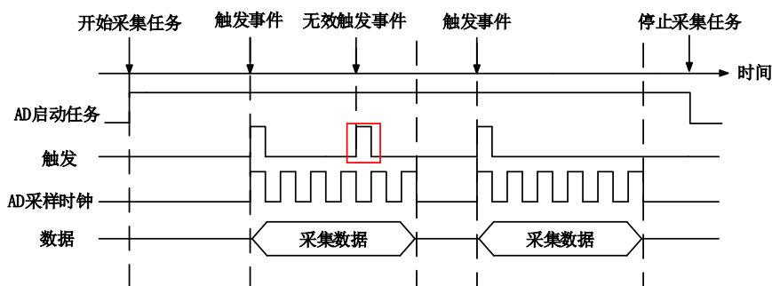
图 4-7-6 重触发
