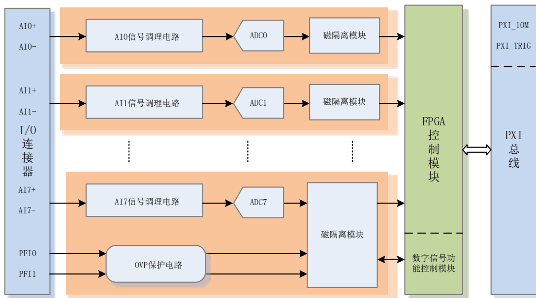
图2-2-1 PXI576X系统框图
