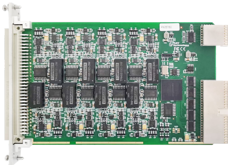
图 3-1-1 PXI576X 正面图
