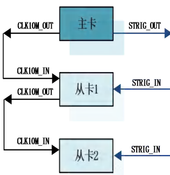
图 4-10-1 主从卡级联
