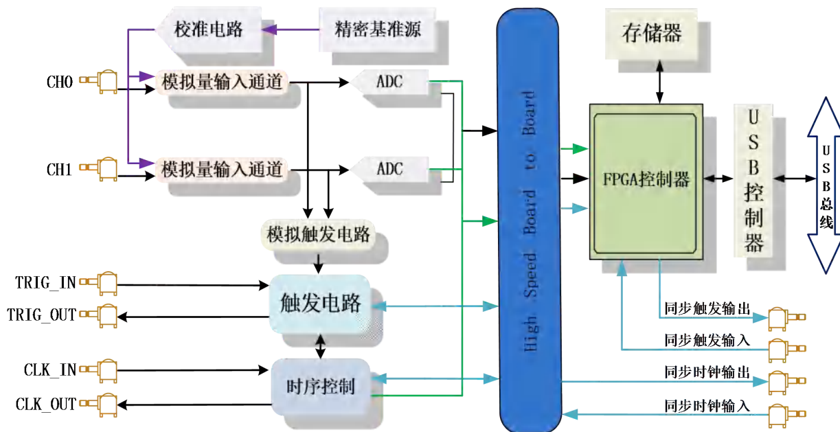
图 3-1-1 USB8914\8912 系统框图
