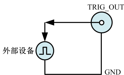
图 4-8-10 触发信号输出连接
