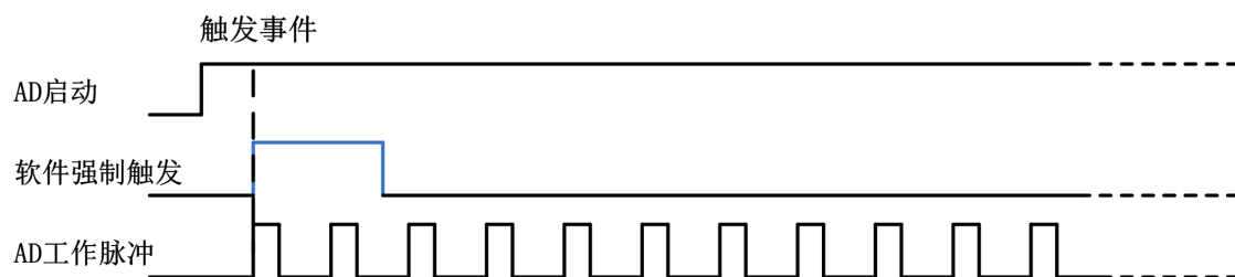
图 4-8-3 AD 软件触发
