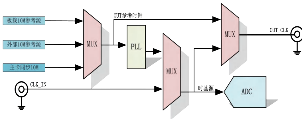
图 4-7-1 时基源框图
