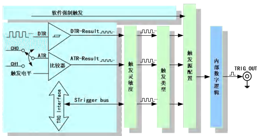
图 4-8-1 AD 触发功能框图
