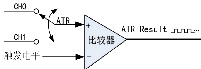
图 4-8-5 比较器
