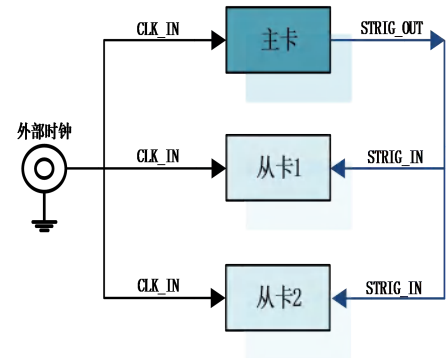
图 4-10-2 采用共同外时钟
