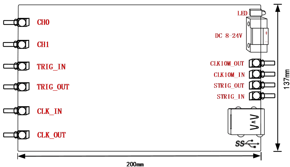
图 3-2-1 USB8914\8912 板卡尺寸图
