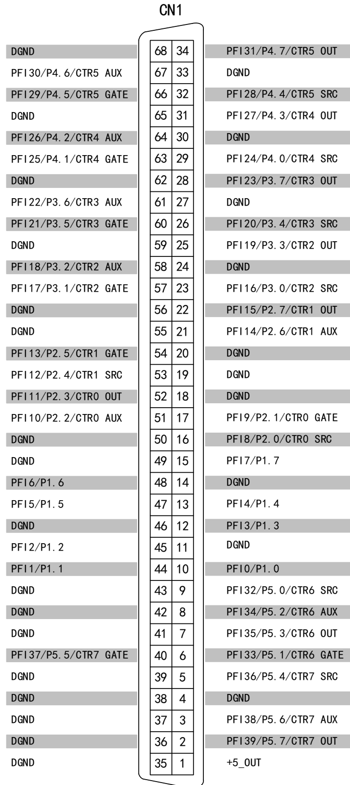
图 3-2-2 PCI2383 接口定义
