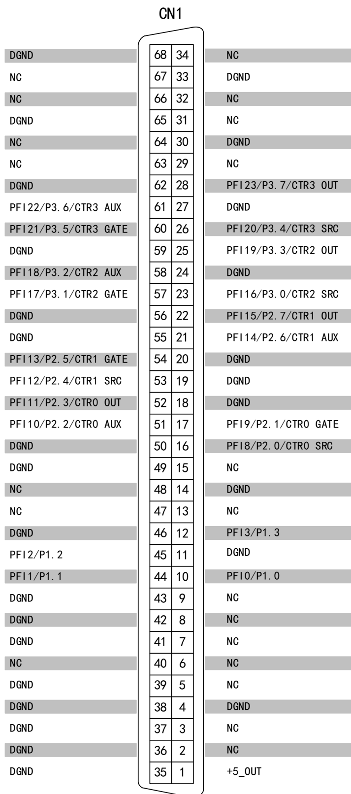
图 3-2-1 PCI2381 接口定义
