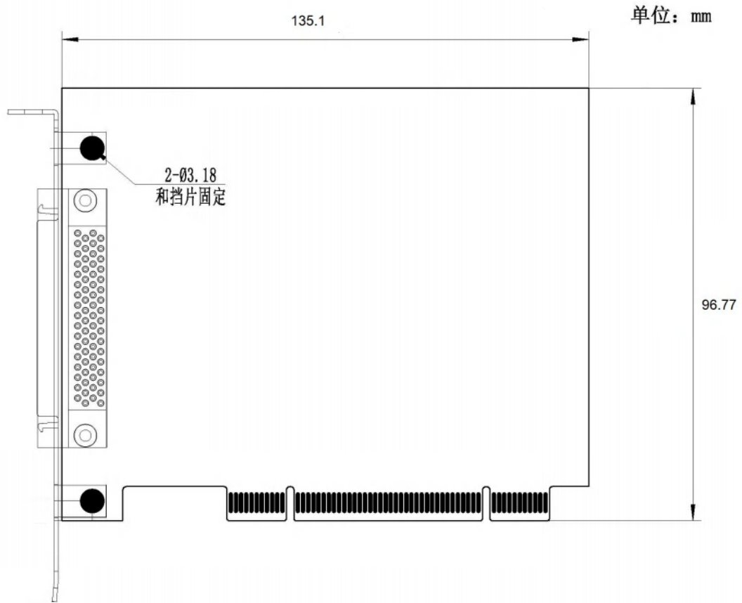
图 3-3-2 PCI238X 板卡尺寸图
