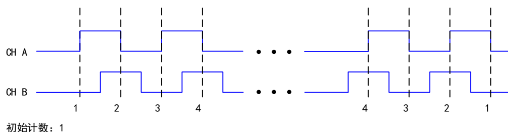
图 4-7-2 X2 编码
