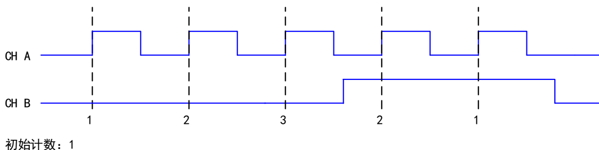
图 4-7-5 单脉冲编码
