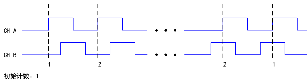
图 4-7-1 X1 编码
