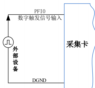
图4-8-9 数字触发连接方法
