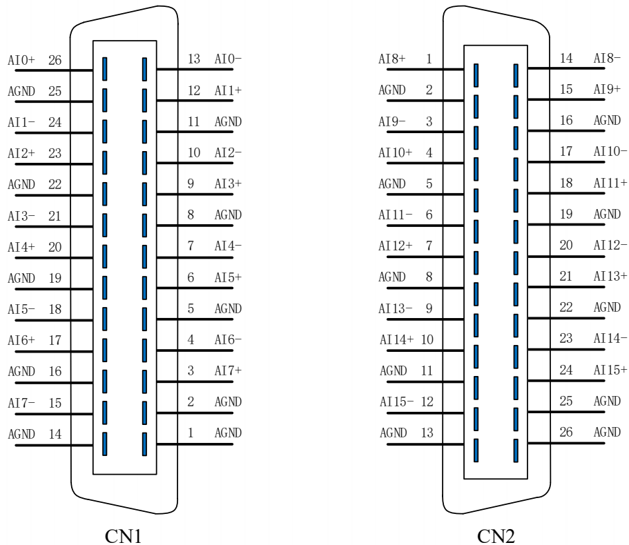
图 3-3-1 8816 接口定义
