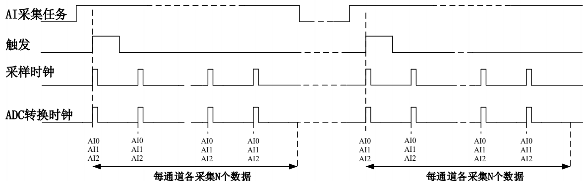
图4-6-2 有限点采样
