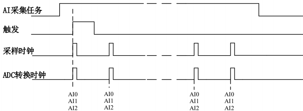
图4-6-3 连续采样
