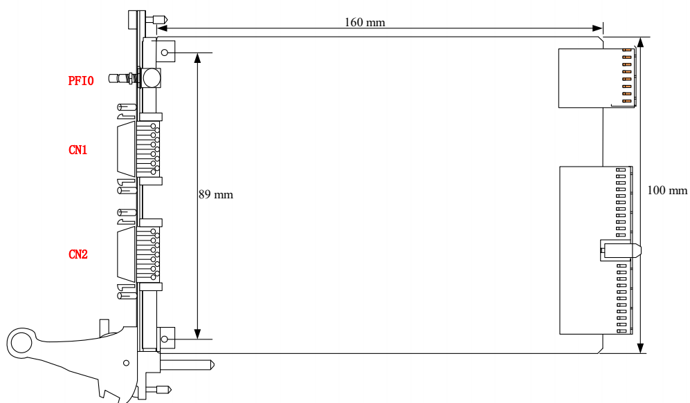
图 3-2-2 PXI8816 板卡尺寸图
