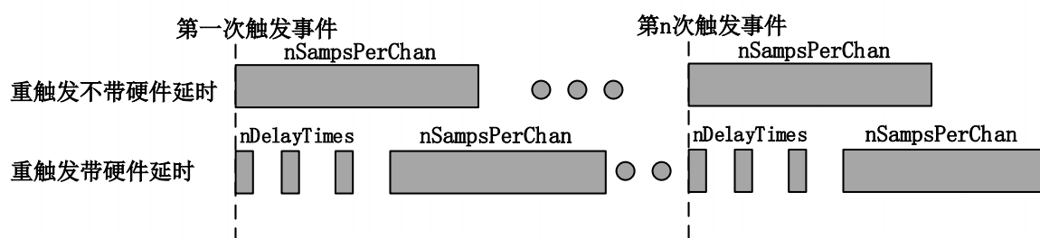
图 4-7-5 AI 重触发
