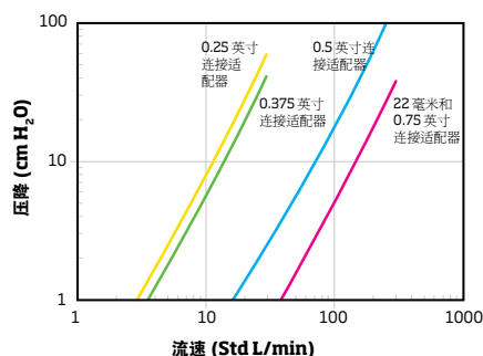
5000 系列压降
