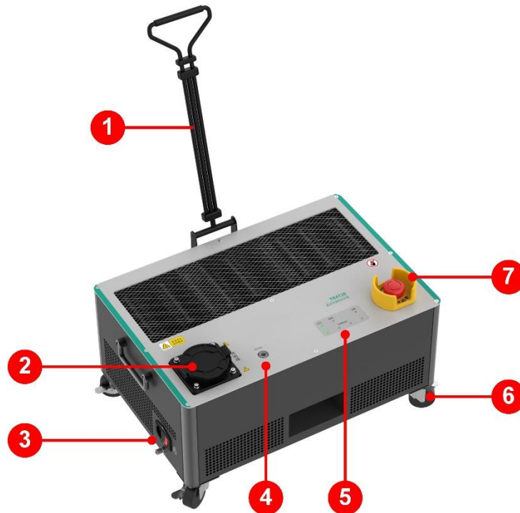
☆ TK4710-20kW 仪器前面板
