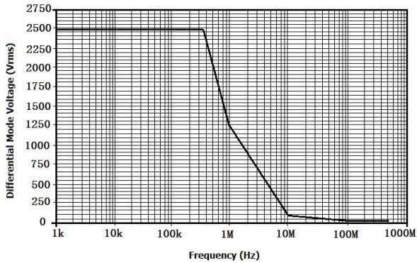
图 3 DPX6350B 最大差模电压 VS 频率
