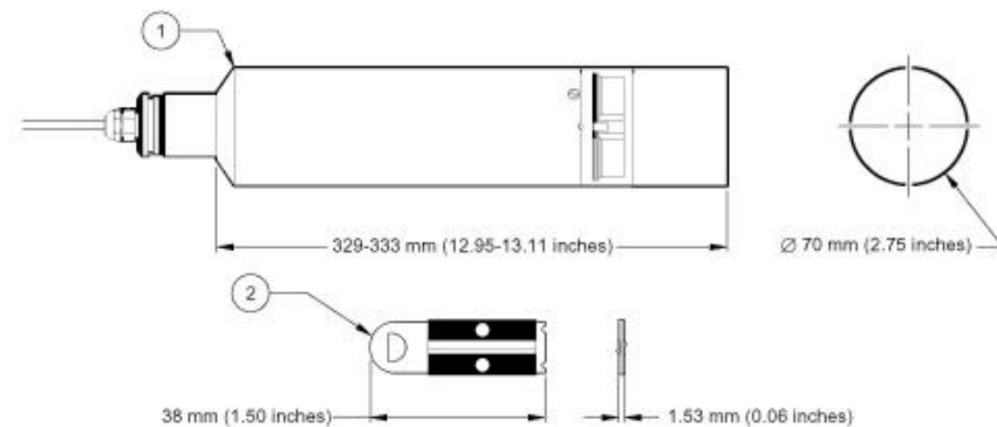
图 3 传感器部件
