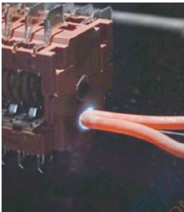
图 B.2 蓝晕在灼热丝顶部的示例
