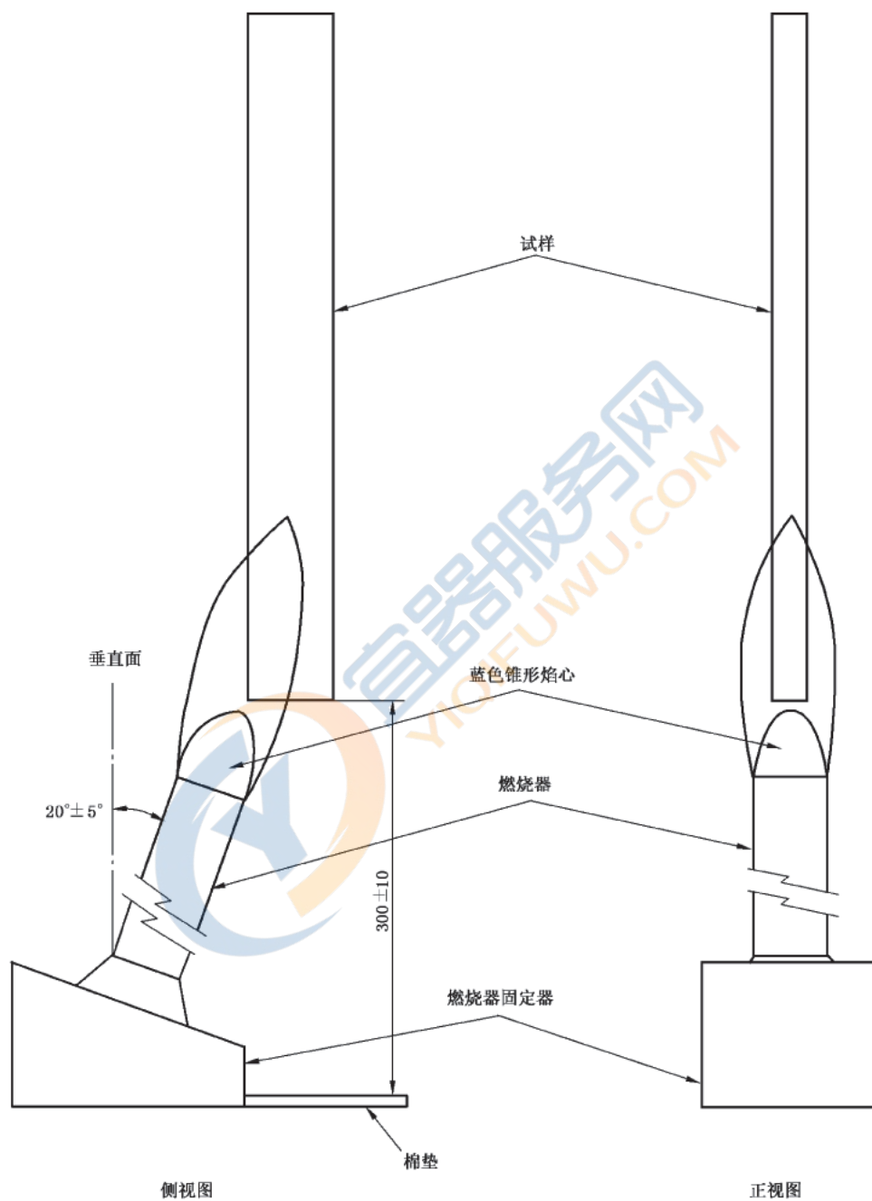
图 1 条形试样的垂直燃烧试验
