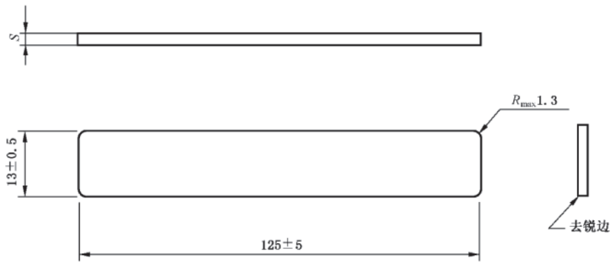
a) 条形试样
