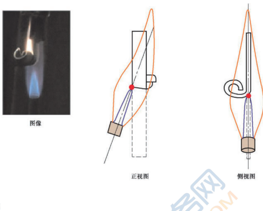
图 A.3 对卷起的试样的火焰施加点
