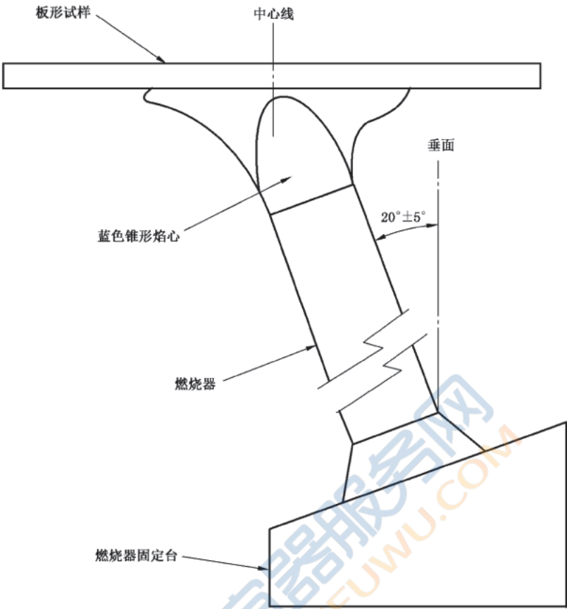
图 2 板形试样的水平燃烧试验
