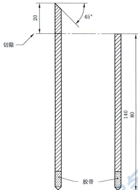
图4 轧制的试样
