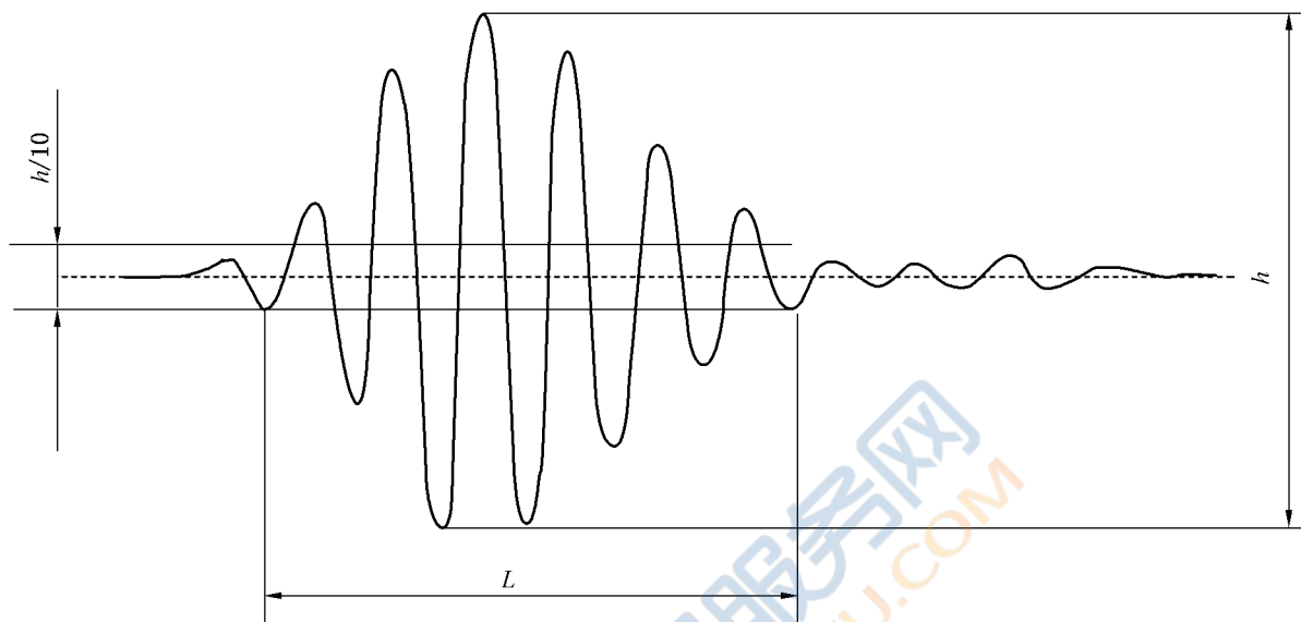
图 2 典型的脉冲波形示意图
