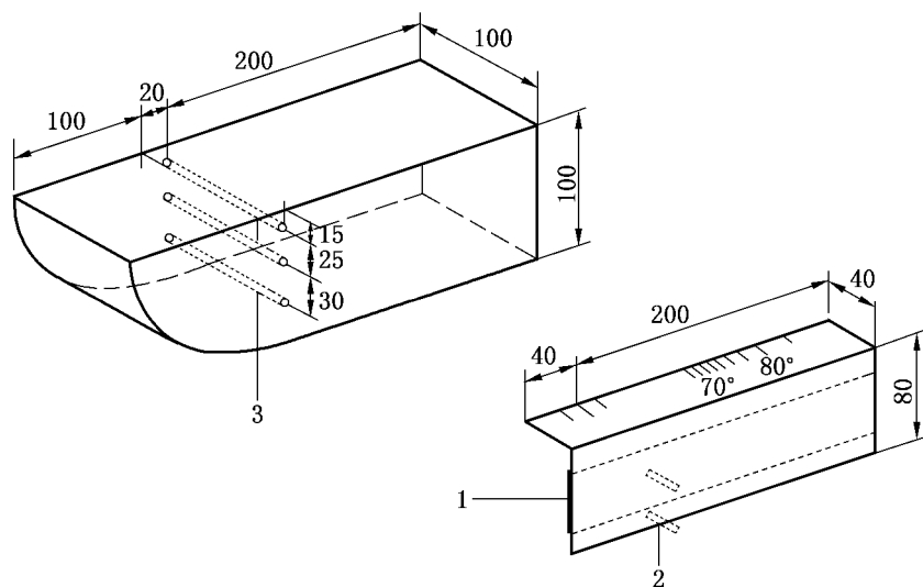
图3 带有活动标尺的斜探头校准试块
