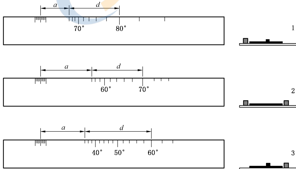
图4 装在斜探头校准试块上的 L 型标尺
