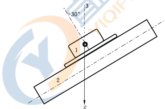
图4 -30^\circ 测量位置的加速度计安装结构示意图
