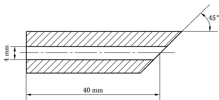
图1 标准气阻
