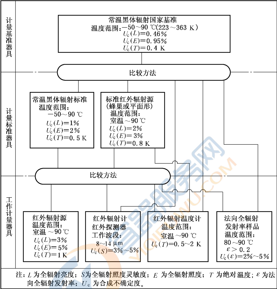
四 常温黑体辐射计量器具检定系统框图
