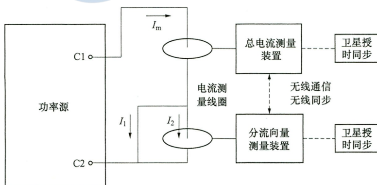
图 A.1 主从模式工作原理
