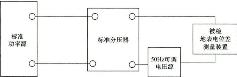
图 7 地表电位差测量误差和抗干扰试验接线图
