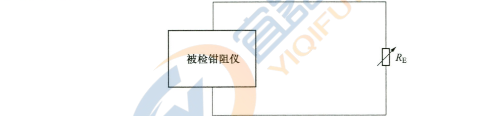
图 4 钳表法测试仪示值误差试验接线图
